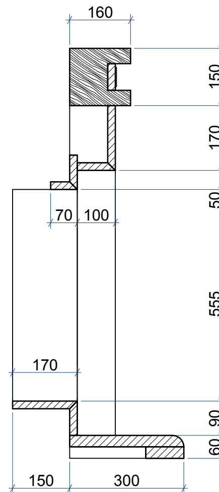
Сечение 2-2
