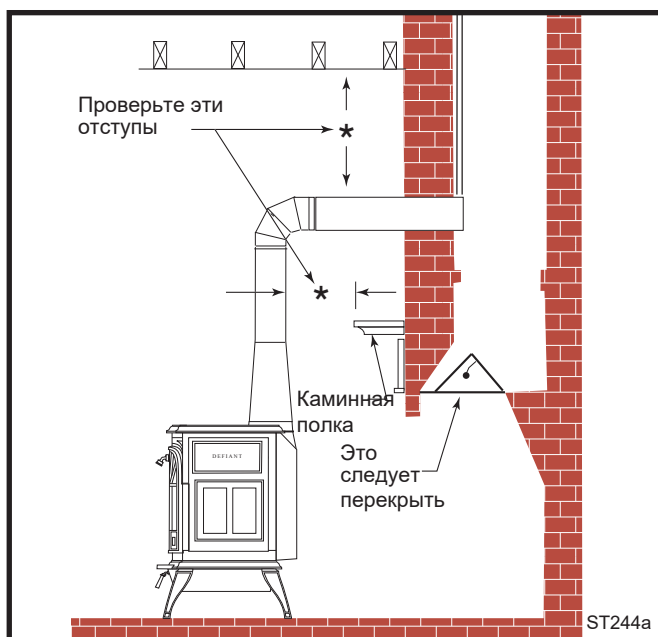
Рис. 8 При таком расположении соединительная труба крепится к дымовой трубе над каминным отверстием.
