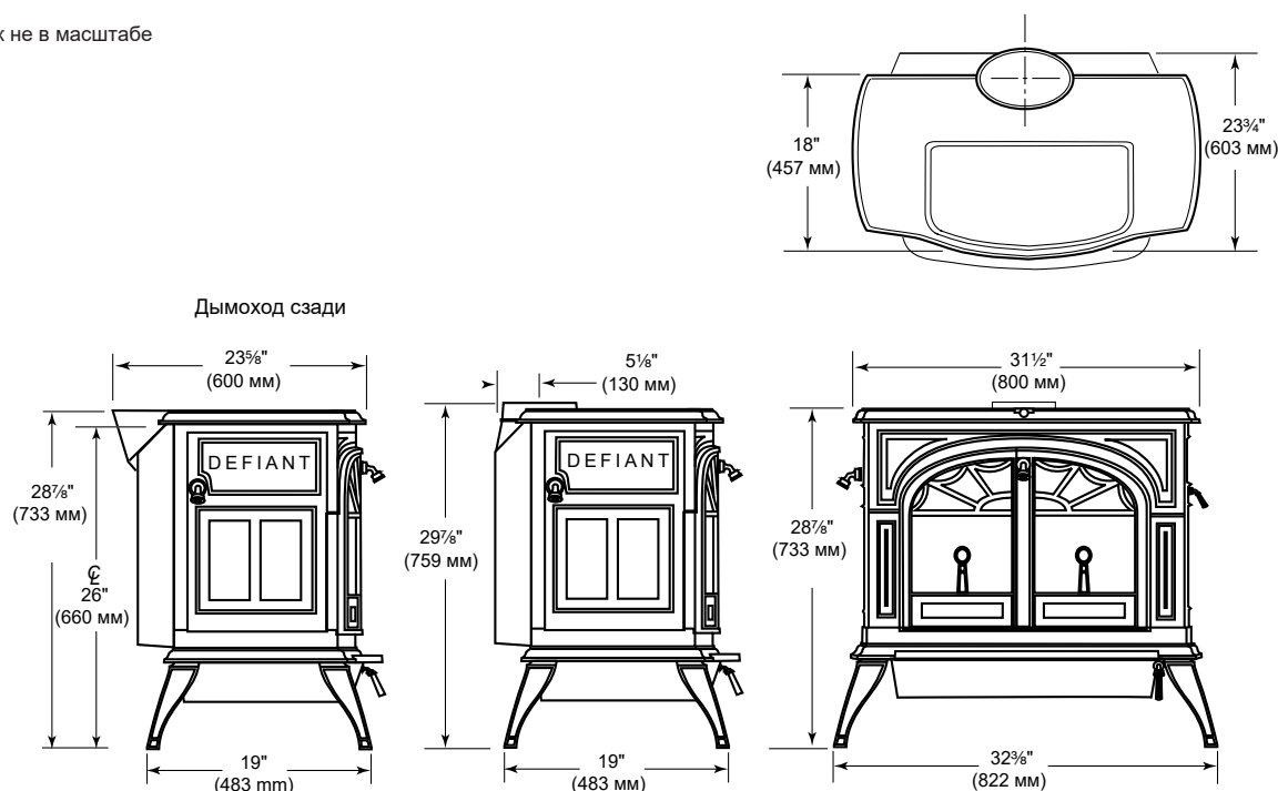
Рис. 1 Размеры печи Defiant 1975
