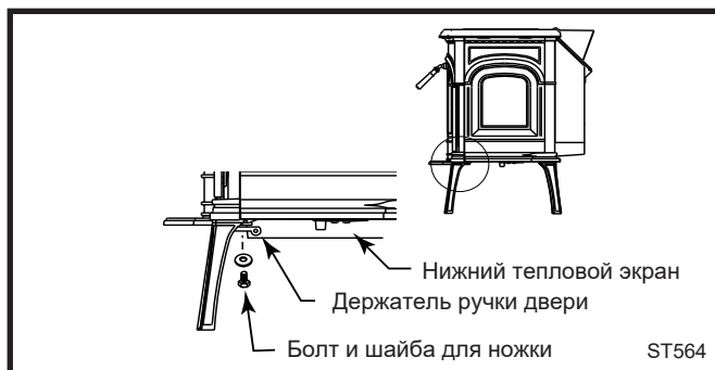
Рис. 21 Положение держателя ручки и теплового экрана.
