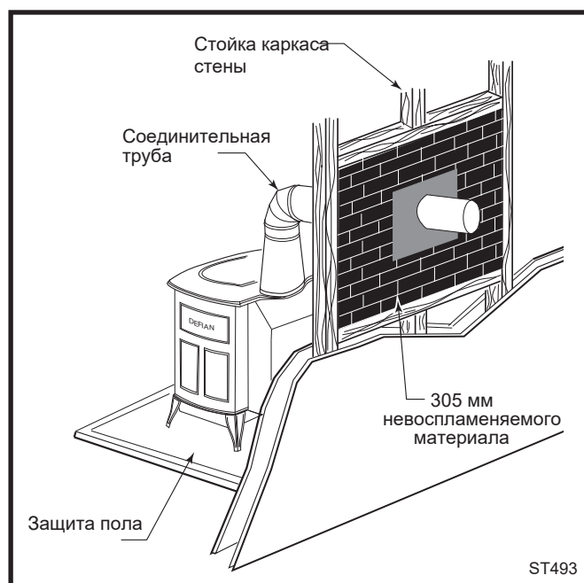
Рис. 10 Одобренный метод пропуска через стену.
