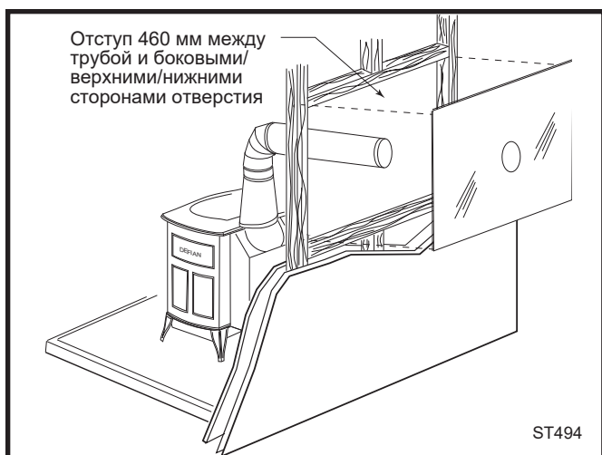
Рис. 11 Одобренный в Канаде пропуск через стену
