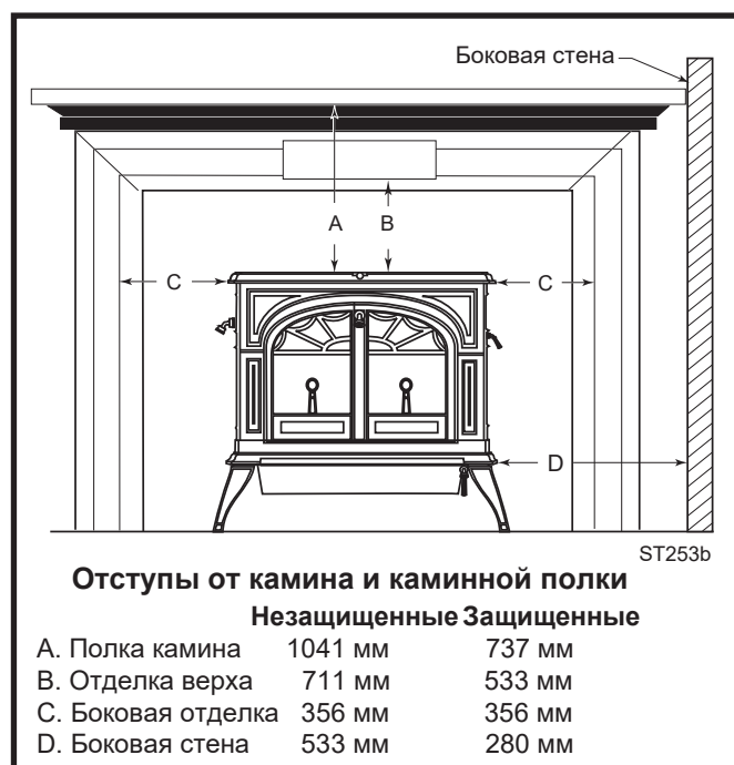
Рис. 15 Оставляйте отступы до воспламеняемых компонентов каминной облицовки
