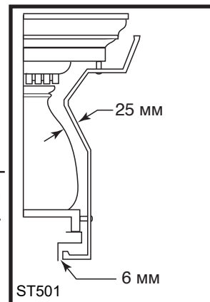
Рис. 14 Экран для каминной полки.
