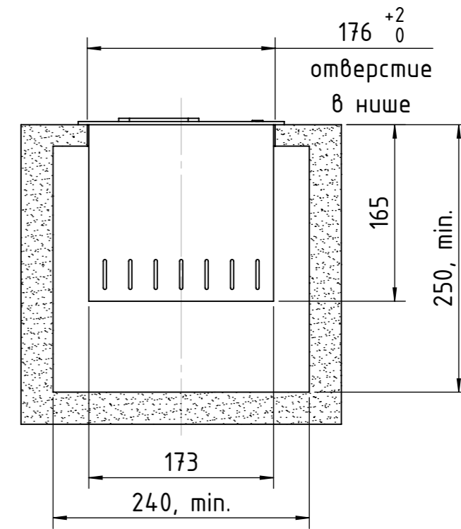
Y-Y (1 : 5)
